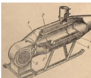
Рис. 170. Теплогенератор ТГ-150:
