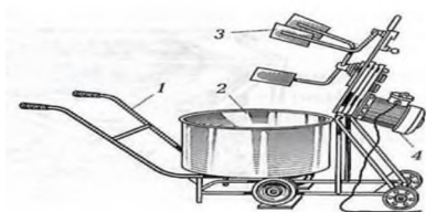
Рис. 5.2. Растворосмеситель: СО-23В: 1 – тележка; 2 – смесительный барабан; 3 – лопасть; 4 – электродвигатель
