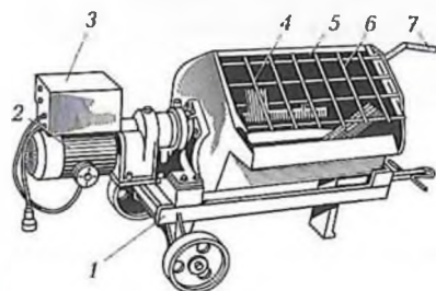
Рис. 5.1. Растворосмеситель: СО-46Б:
