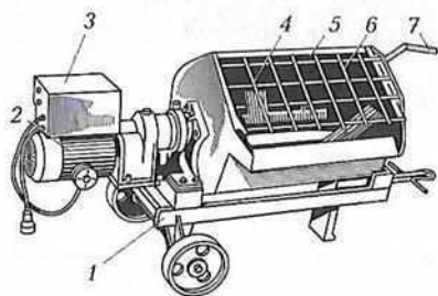
Рис. 5.1. Растворосмеситель: СО-46Б:
