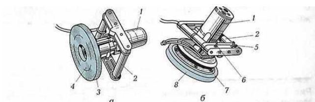
Рис. 5.15. Штукатурно-затирочные электрические машины: а — СО-86А; б — СО-112А; 1 — корпус электродвигателя; 2 — ручка; 3, 4 и 8 — затирочные диски; 5 — электровыключатель; 6 — регулятор подачи воды; 7 — резиновая подвеска
