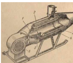
Рис. 170. Теплогенератор ТГ-150:
