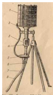
Рис. 171. Горелка ГК-1-50:
